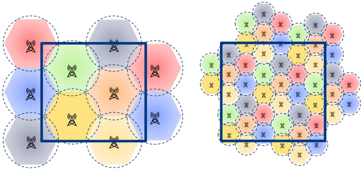
Figuur 1: Door gebruik te maken van kleinere cellen en lagere zendvermogens kan dezelfde radiofrequentie vaker worden hergebruikt. Gevolg is dat op dezelfde oppervlakte zonder nieuwe frequentiebanden in te zetten veel meer capaciteit kan worden aangeboden en dus meer gebruikers met hogere snelheden kunnen zenden en ontvangen (Stratix).
